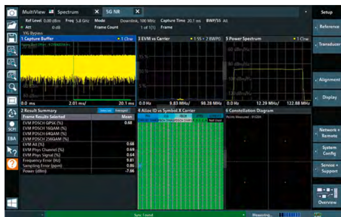
R&S®FSV3-K144 (ダウンリンク) および R&S®FSV3-K145 (アップリンク) オプションによる、5G NR信号の解析。
